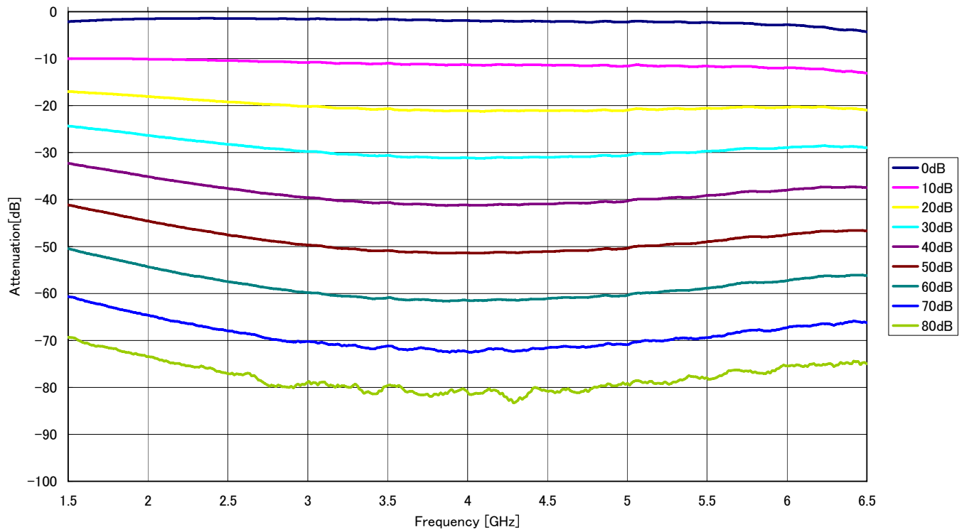
MAT800 Model D Attenuation(S21)
