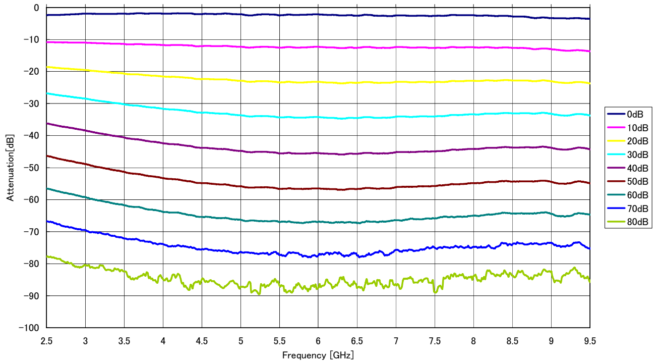
MAT800 Model B Attenuation(S21)
