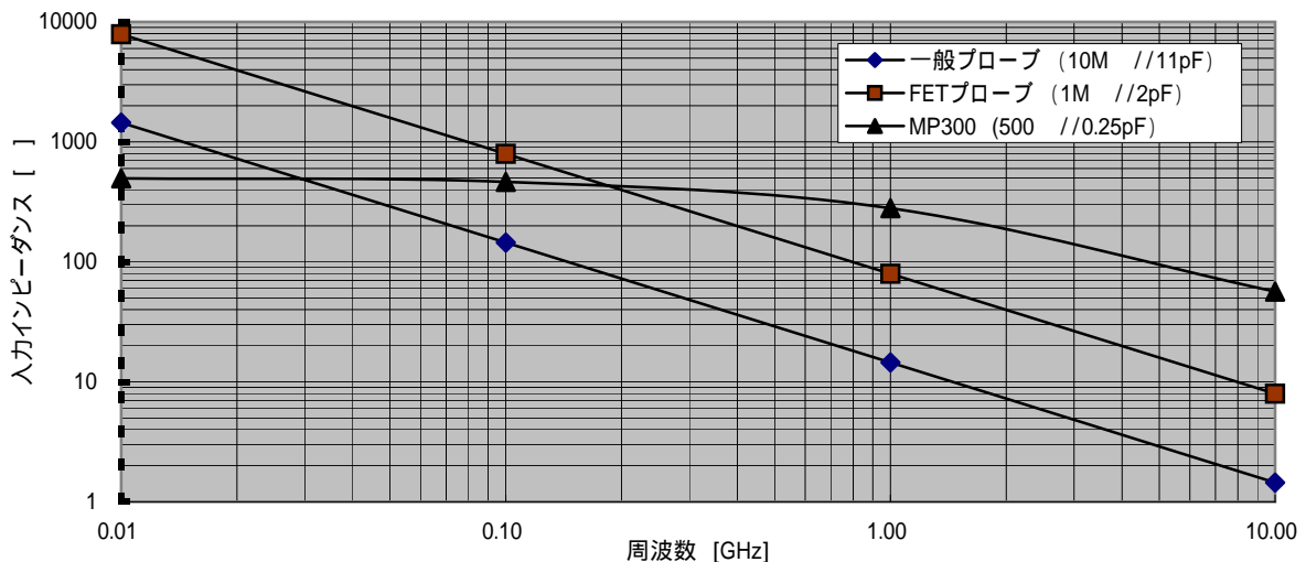
入力インピーダンス(特性例)
